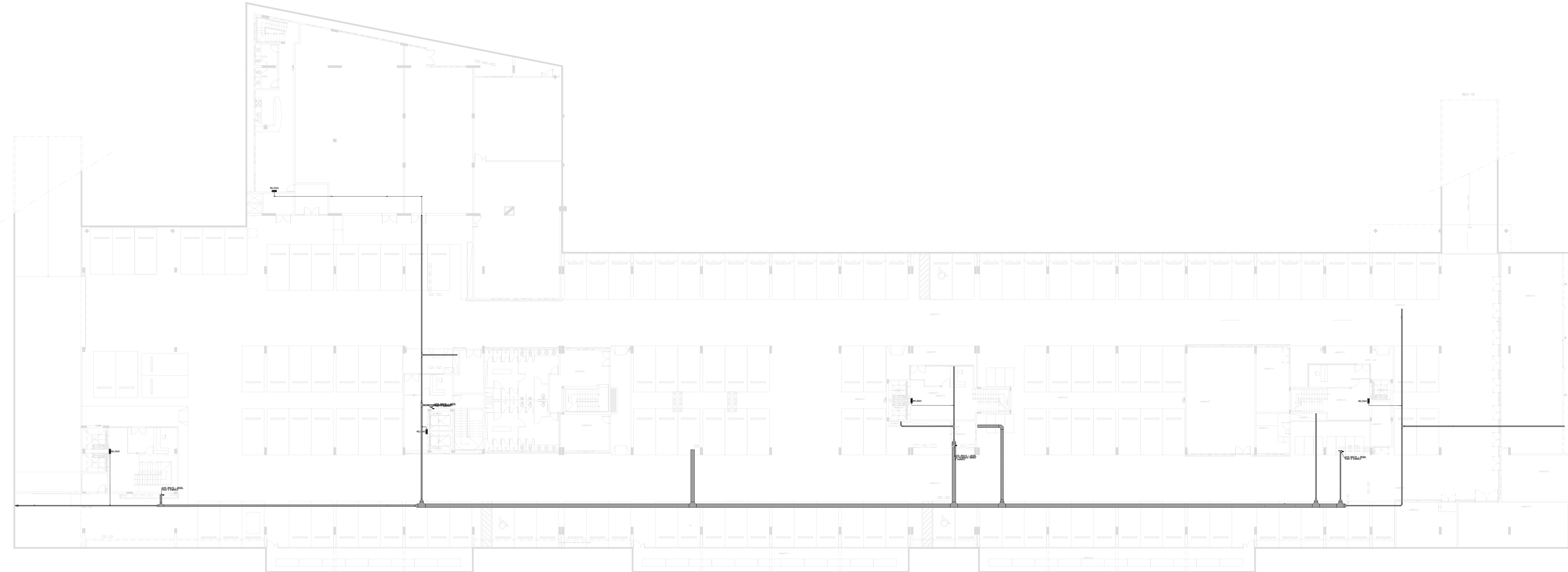
1 PLANTA BAIXA DO SUBSOLO ESC 1/200
